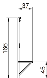
TIPOLOGIA E2 Panca singola a muro con seduta e schienale alto con appendiabiti.
